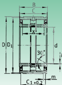
SL0450..-PP SL04..-PP
