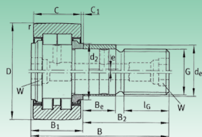
NUKRE PWKRE..-2RS
