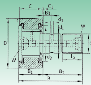
KRV..-PP
