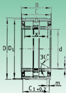
SL0450...-PP SL04...-PP
