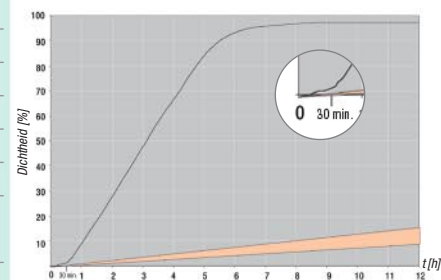
Uithardingstijd van Terostat 8630 2K HMLC in vergelijking met andere 1K producten
