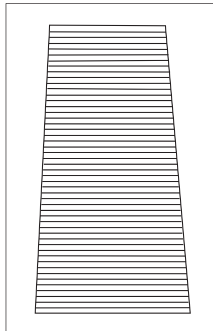
Meetekegel 4 Meetbereik 151 tot 200 mm Oplopend per mm Hoogte 375 mm Bodemplaat afneembaar
