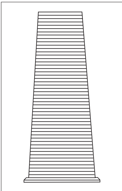
Meetekegel 3 Meetbereik 101 tot 150 mm Oplopend per mm Hoogte 375 mm Bodemplaat afneembaar
